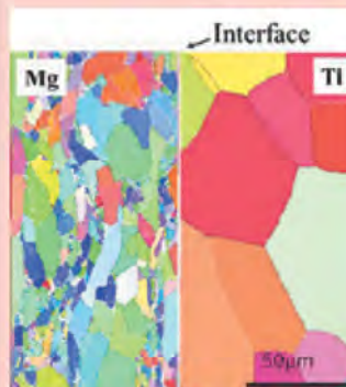
チタン/マグネシウム焼結接合材の 生分解性評価
