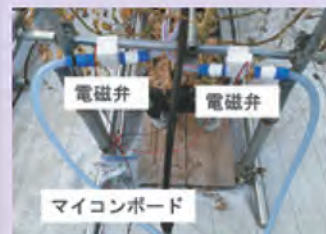
図3 トマト栽培における自動灌水システムの構築に関する研究
