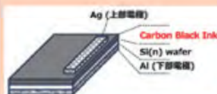
短 TAT プロセス型新型太陽電池の 試作品（上）と構造図（下）
