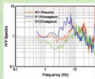
図3 H/Vスペクトル
