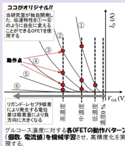
図3 新規バイオセンサの開発例
