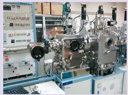
図4 真空蒸着－グローブボックスー貫装置 (ALS テクノロジー製 ほか)
