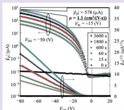
図1 酸化銀を電極上を持つ有機FETの伝達特性
