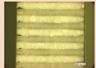
図2 レーザーの加工孔
