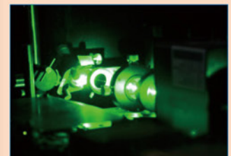
図3 Nd 3+ :YVO 4 ピコ秒レーザー
