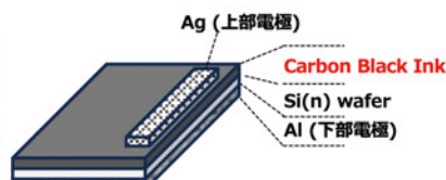
短TATプロセス型新型太陽電池の試作品(左)と構造図(右)
