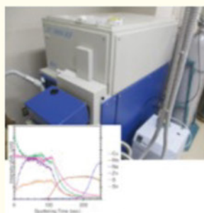
材料中の元素の深さ方向分布を 可視化する GD-OES
