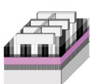
CZTS薄膜太陽電池試作品(左)と構造図(右)
