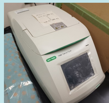
PCR
