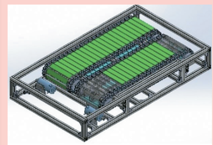
図4 不意な滑り再現トレッドミル
