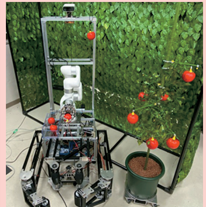
図7 ポット栽培野菜収穫ロボット
