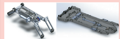
図3 橋梁遊間部の打音点検装置
