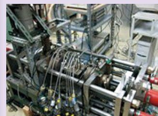
図3 背圧付加型溶融樹脂流動試験機
