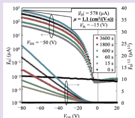
図1 酸化銀を電極上に持つ有機FETの伝達特性
