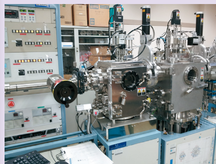
図4 真空蒸着ーグローブボックスー貫装置 (ALSテクノロジー製 ほか)
