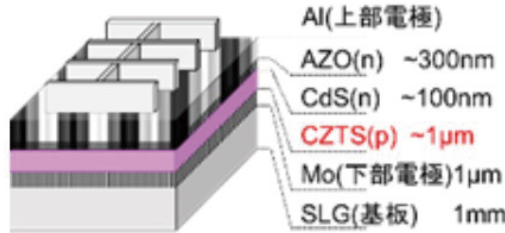
CZTS 太陽電池の構造図
