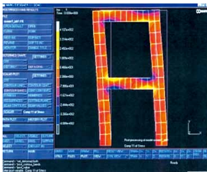
有限要素法による2層ラーメン構造の解析 FEM Analysis on 2-story Viaduct
