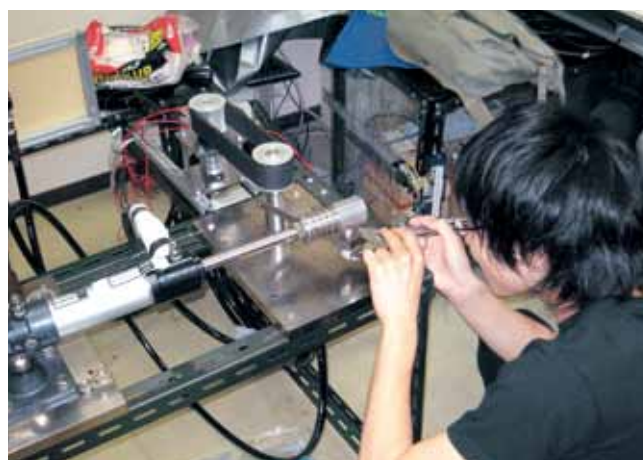
小型船舶における舵角システムに関する研究 Study on Rudder Angle Servo System for Pleasure boats
