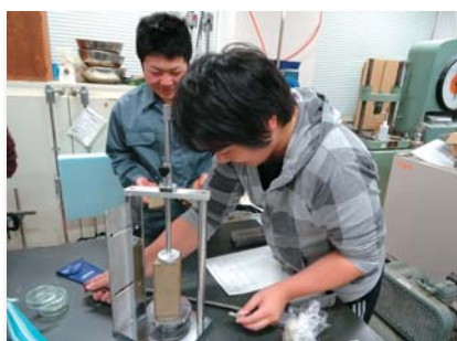
土質実験 (4学年) Soil Experiment (4th grade)
