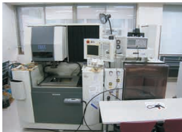
ワイヤ放電加工機 Wire Electrical Discharge Machine
