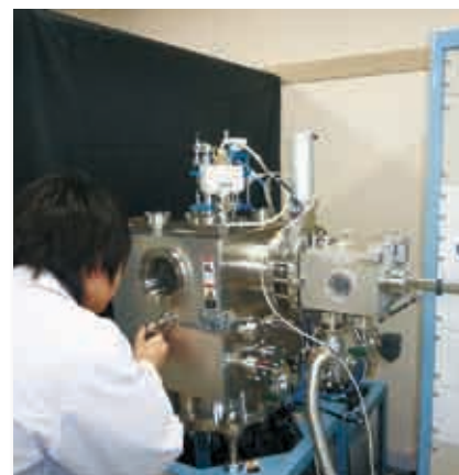
モバイル端末ディスプレイ向け有機EL素子の作製実験 Development of OLED Device for Mobile Terminal's Display
